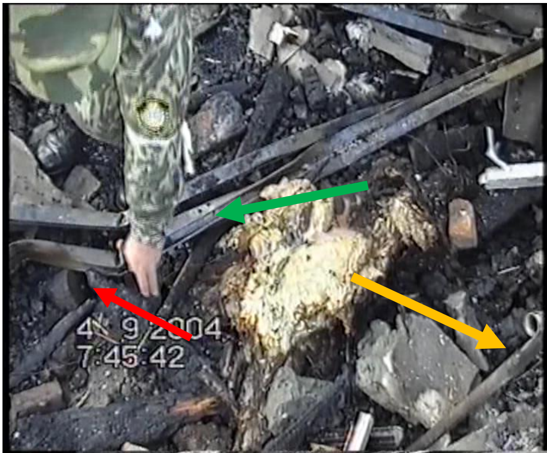
Рис. 83. ОМП. Красной стрелкой указан корпус неразорвавшегося СВУ на базе ОЗМ-72, оранжевой – труба батареи, зелёной – провод к электровзрывателю.
